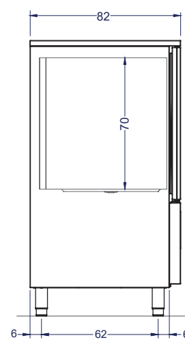
Vista Izquierda
