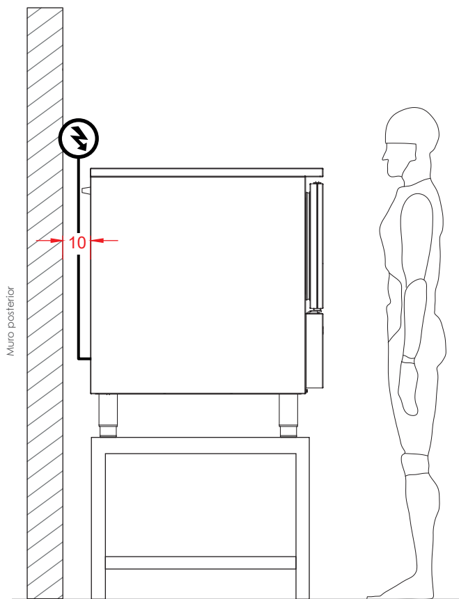
Vista Izquierda
