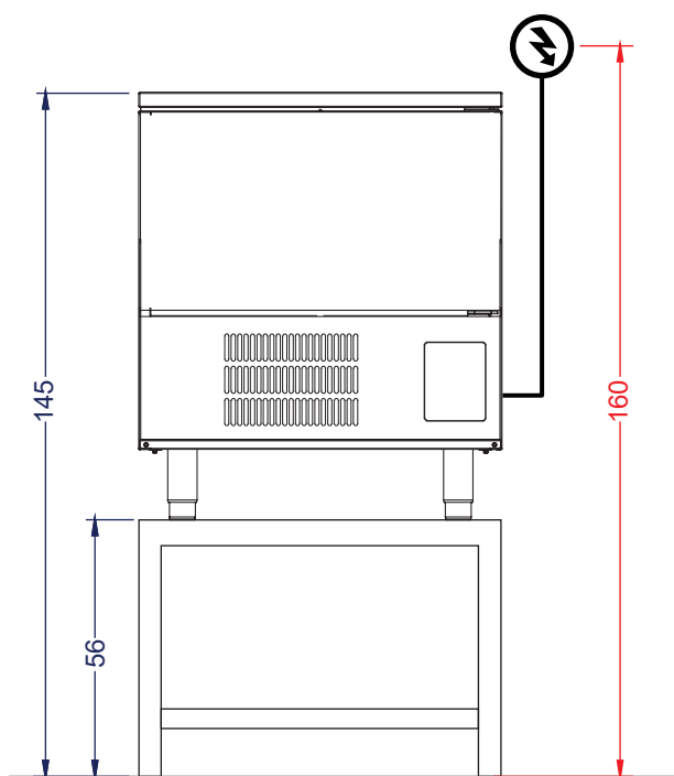
Vista Elevación
