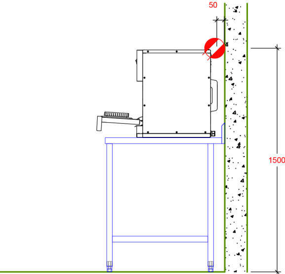
ELEVACIÓN LATERAL
