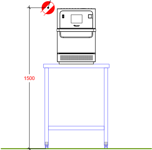
ELEVACIÓN FRONTAL
